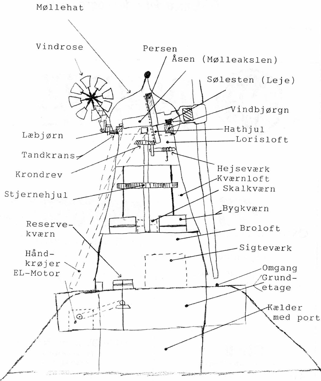
SKITSE OVER SKAMSTRUP LILLEMØLLE:
