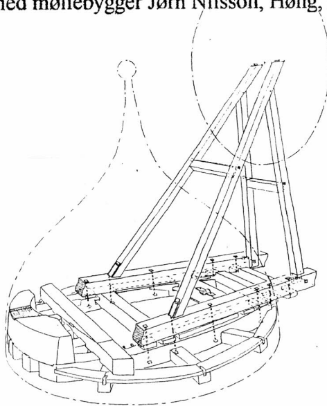
Nye krøjeværksbjælker og stoleværk (1.2.1997 Ole Schneekloth)
